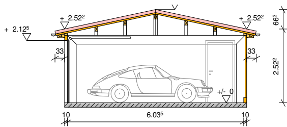
Schnitt A-A
