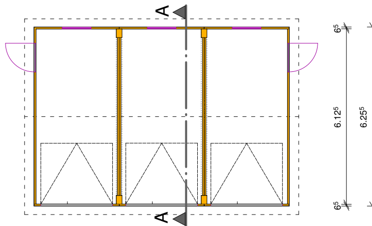
Grundriss
